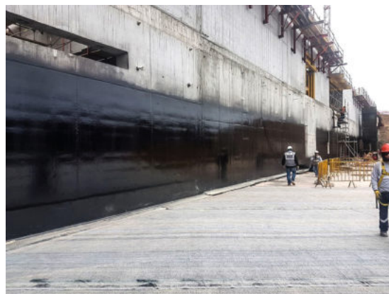
hydroizolace základů (Peru - Muzeum archeologie)
